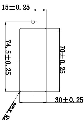
安裝尺寸
