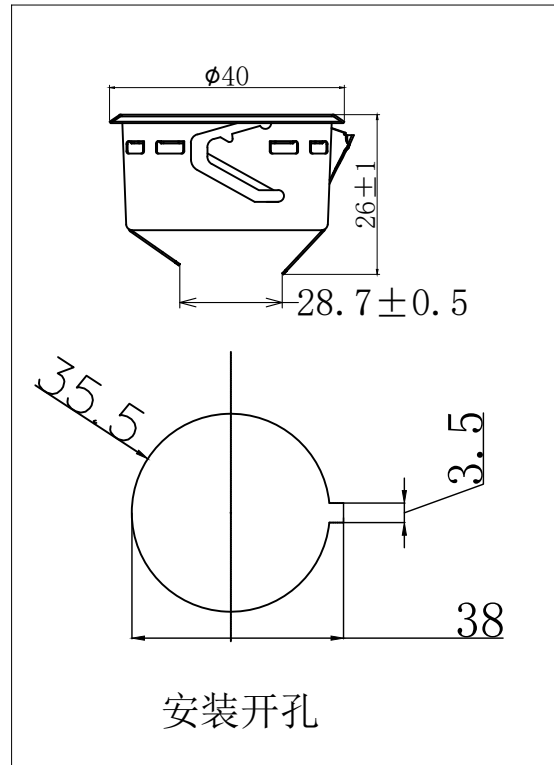
小圆灯壳
