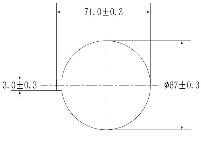
安装开孔
