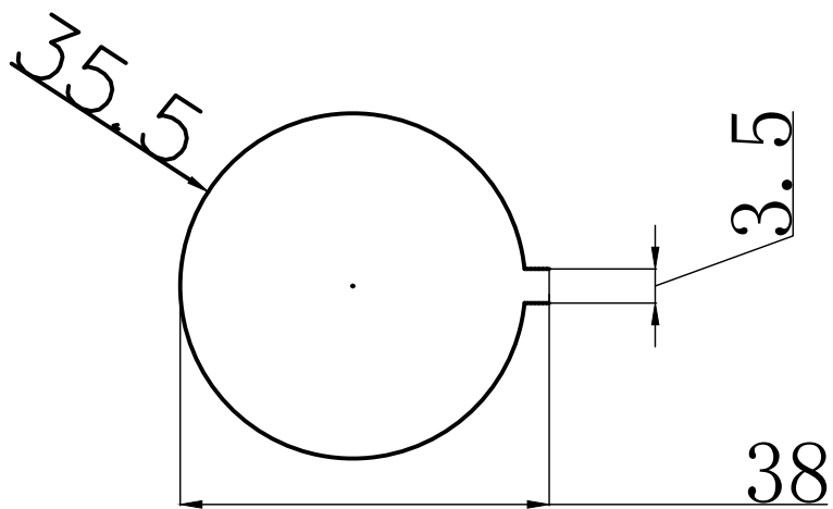
安装开孔
